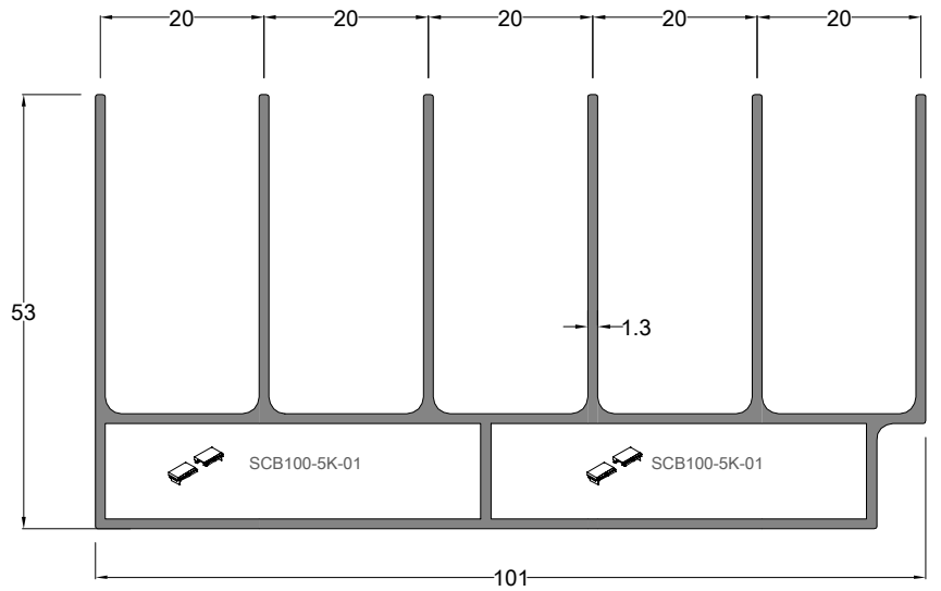
5 Raylı Üst-Yan Kasa Profili TOP-SIDE QUINTUPLE FRAME PROFILE
