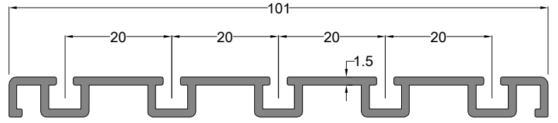
5 Raylı Eşiksiz Alt Ray Profili BOTTOM QUINTUPLE RAIL PROFILE (NON-THRESHOLD)
