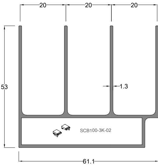
3 Raylı Üst-Yan Kasa Profili TOP-SIDE TRIPLE FRAME PROFILE
