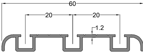
3 Raylı Eşiksiz Alt Ray Profili BOTTOM TRIPLE RAIL PROFILE (NON-THRESHOLD)
