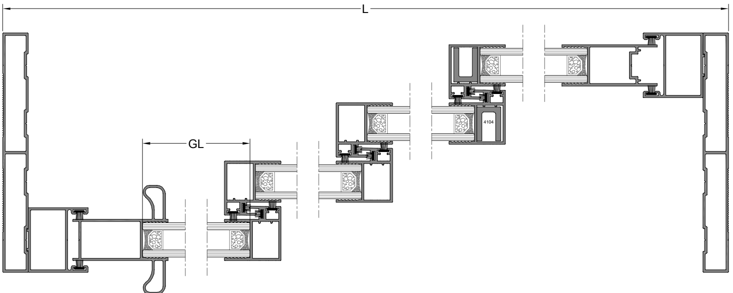
A-A KESİTİ
