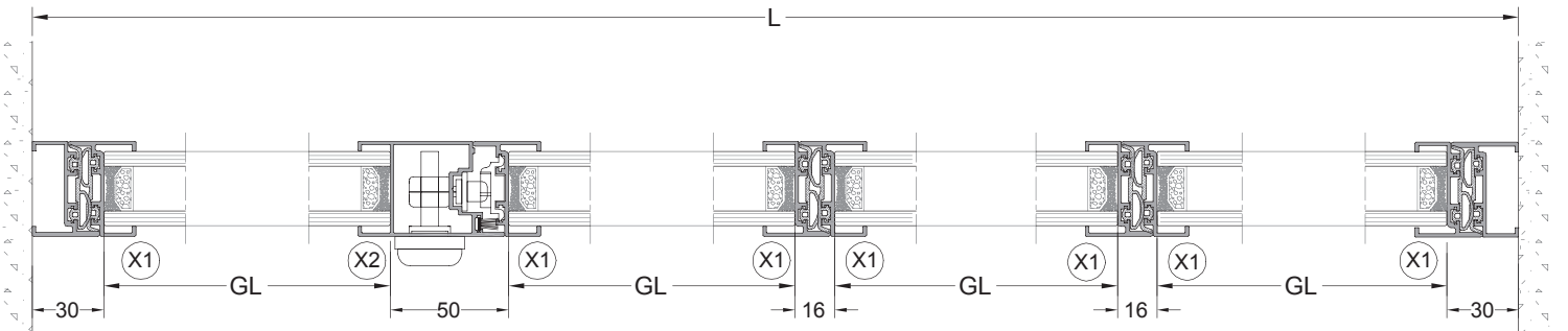
A-A KESİTİ
